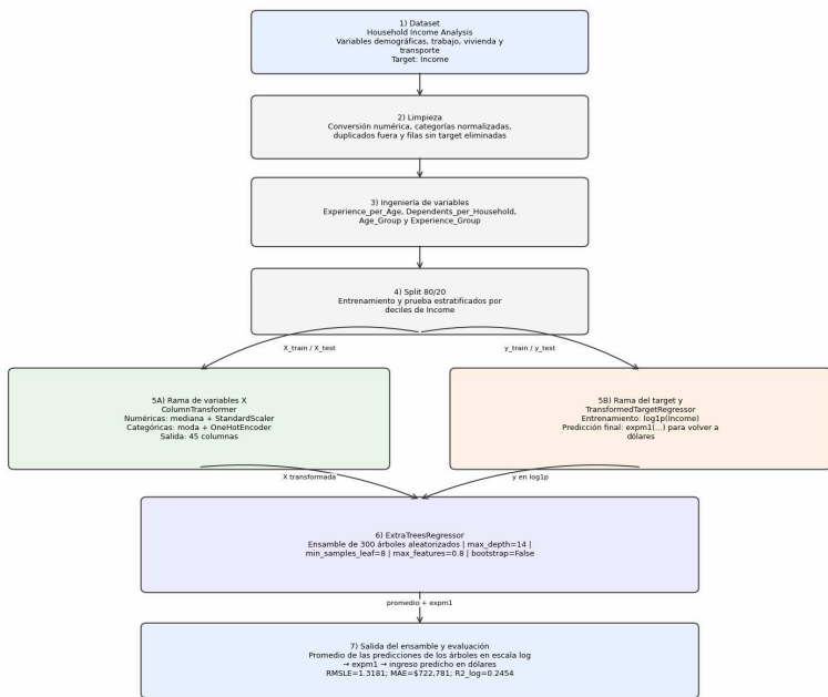
Arquitectura del modelo ganador: Extra Trees
